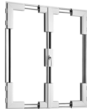
> Battement central ouvrant de 60 mm
