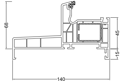
Isolation de 140 mm
