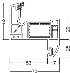
Aile arrondie de 25 mm
