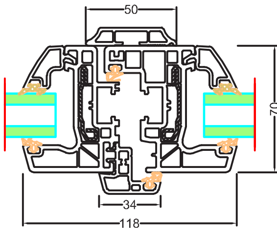
> Battement central ouvrant de 48 mm
