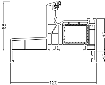
Isolation de 120 mm
