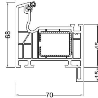
Dormant à recouvrement - Aile de 15
