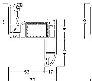
Aile arrondie de 40 mm
