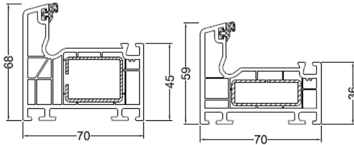
Pose en applique
