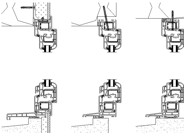
Pose en feuillure
