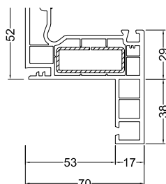
Aile droite de 38 mm
