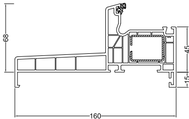
Isolation de 160 mm
