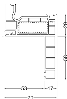
Aile droite de 58 mm
