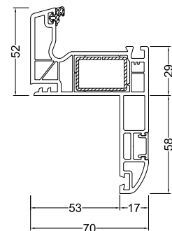
Aile arrondie de 58 mm
