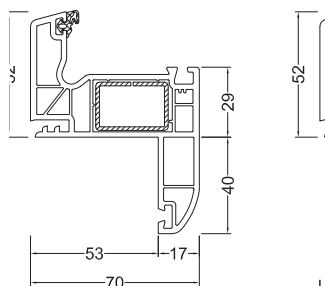
Aile droite de 58 mm
