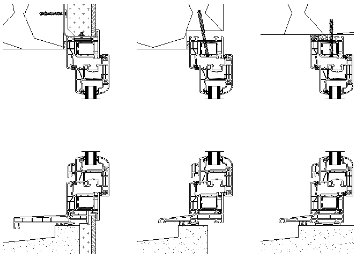
Pose en applique
